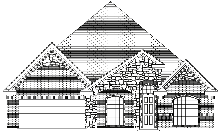
ELEVATION B
