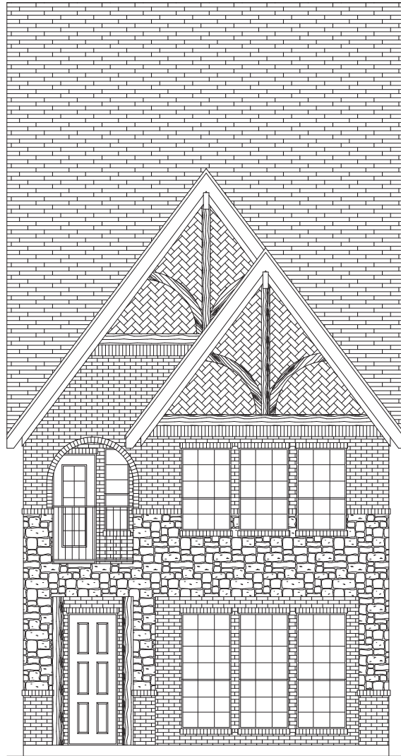
ELEVATION A
