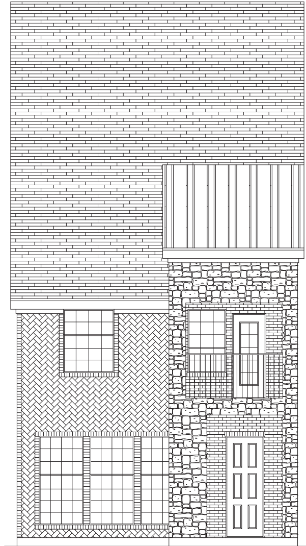
ELEVATION A
