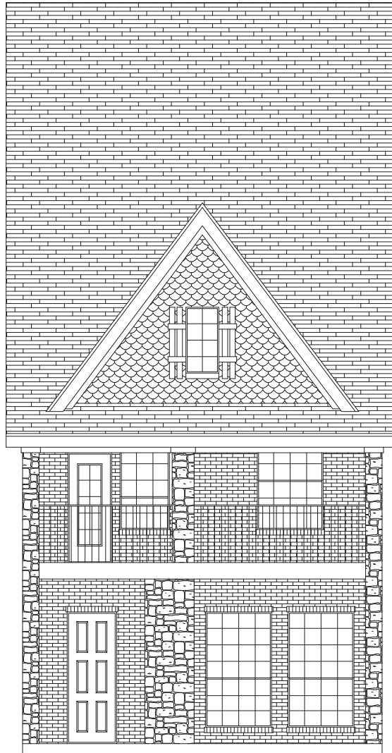
ELEVATION A
